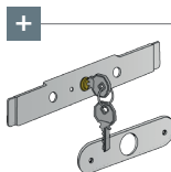
905.30 SERRATURA CON CILINDRO LOCK WITH CYLINDER SERRURE AVEC CYLINDRE
